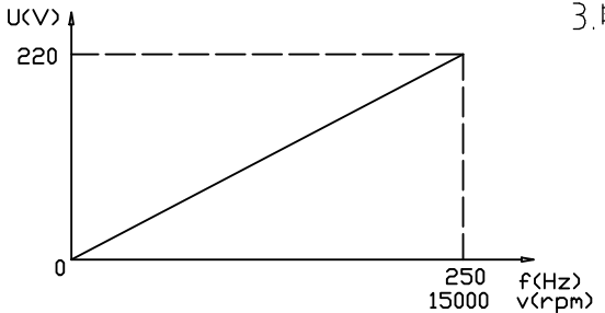
频压曲线
